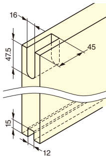
上ローラー用化粧キャップ (P.44) (オプション) を使用する場合
