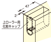
上ローラー用化粧キャップ (P.44) (オプション) を使用する場合
