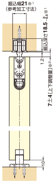
上レール掘込用
