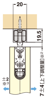
上レール面付用
